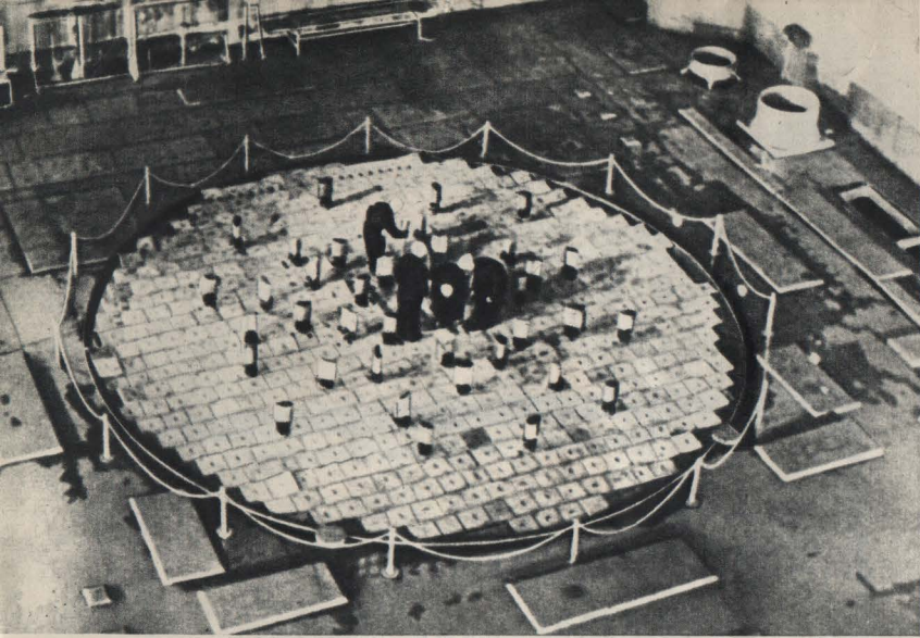
Верхняя часть реактора новой советской атомной электростанции. Первая очередь станции электрической мощностью 100 тысяч киловатт уже вступила в строй. Полная мощность этой крупнейшей в мире атомной электростанции будет доведена до 600 тысяч киловатт.
